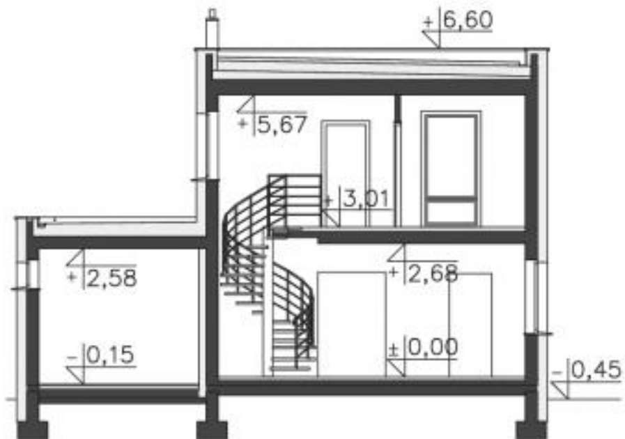
STANDARDTREPPE
